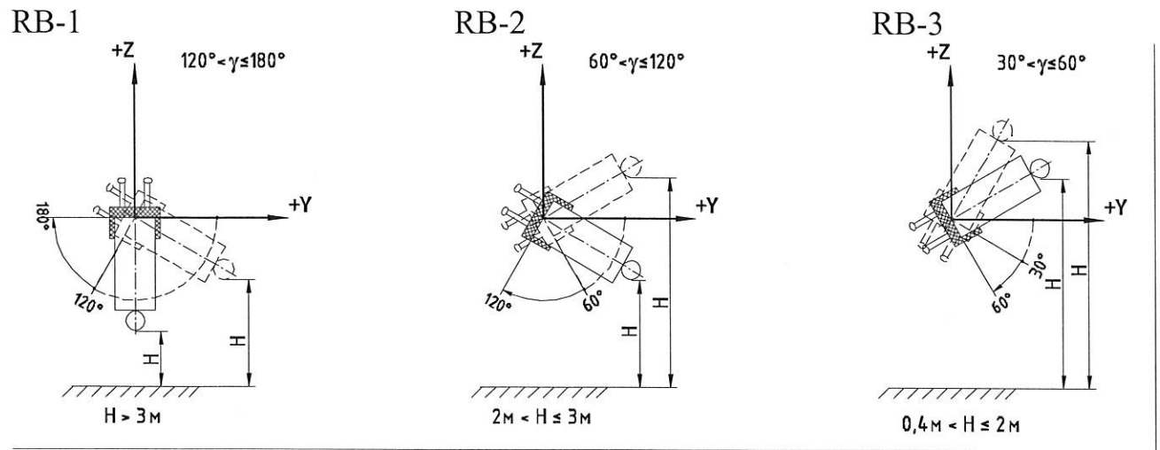
Рис. 3. Наклон пассажирских кресел наборов
